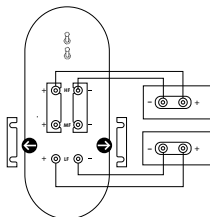
Bi-amp wiring
