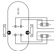
Bi-amp wiring
